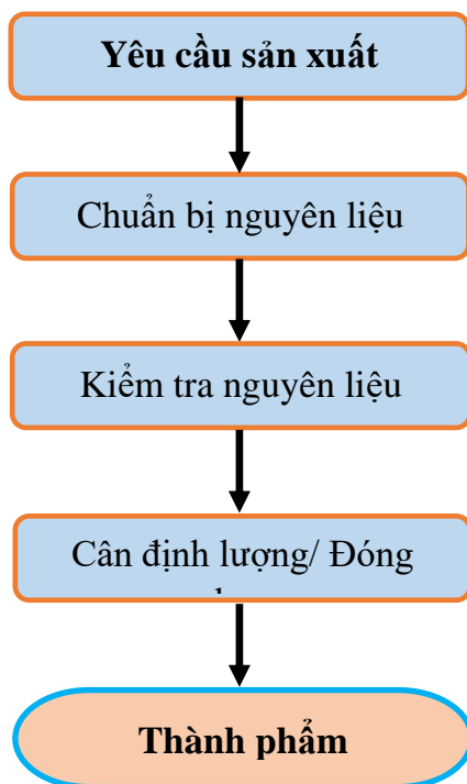
Hình 1.3. Quy trình công nghệ đóng gói phân bón Urê, DAP và Kali
