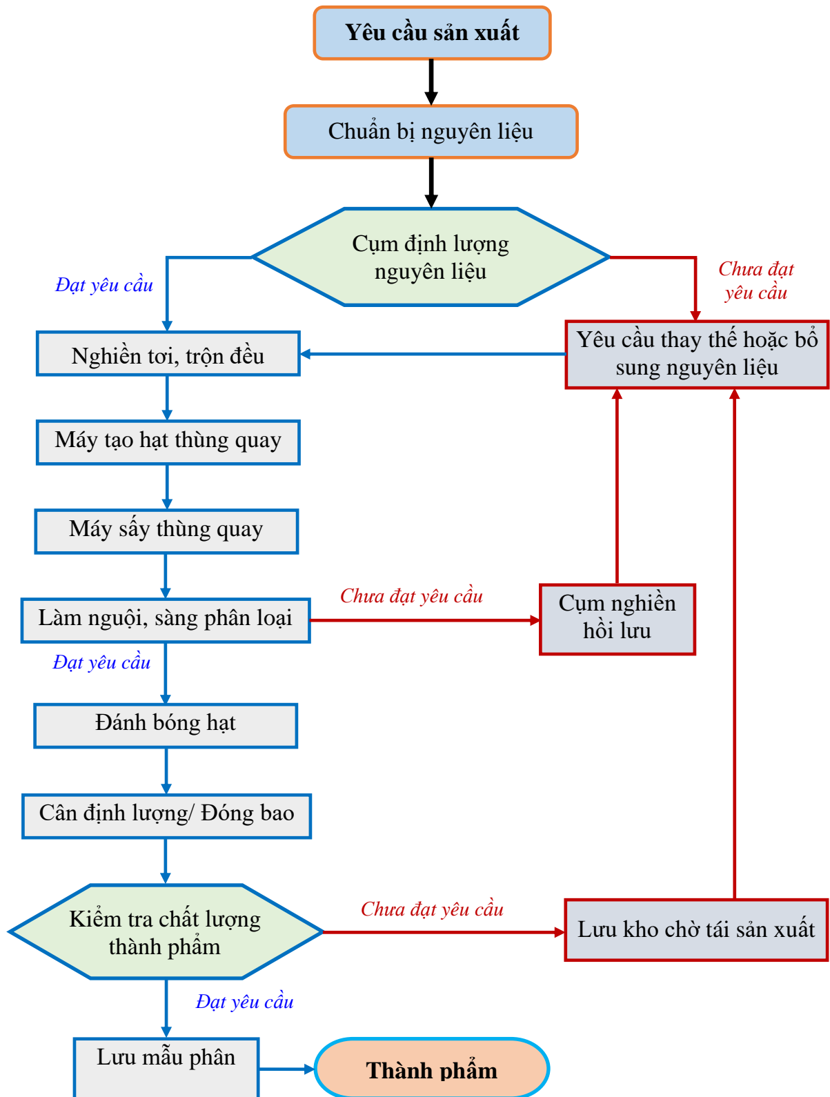
Hình 1.5. Quy trình công nghệ sản xuất phân bón hữu cơ và hữu cơ khoáng
