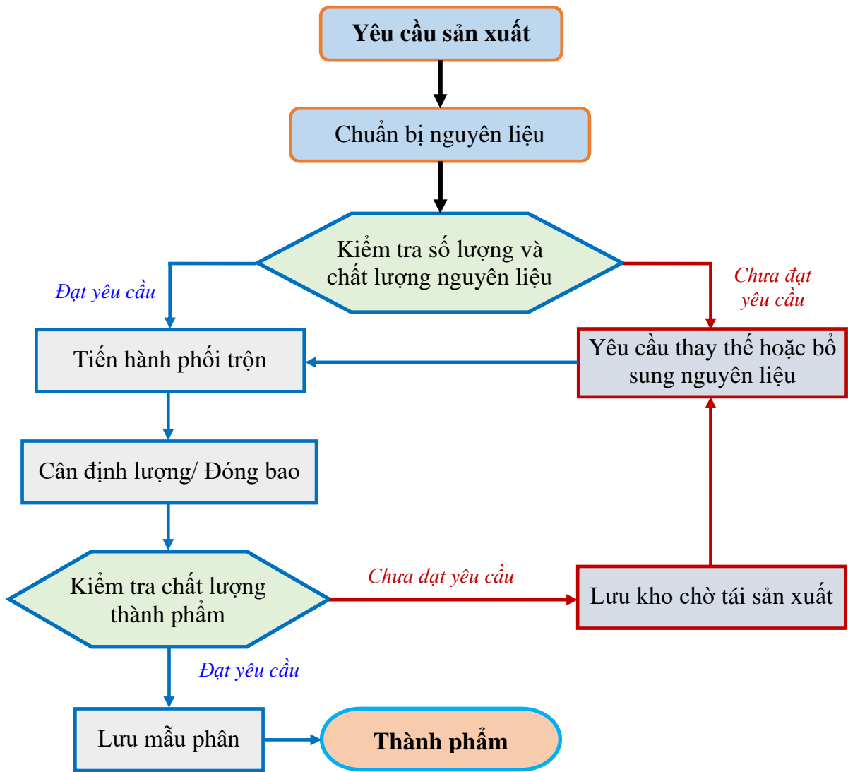
Hình 1.2. Quy trình công nghệ phối trộn phân bón hỗn hợp NPK
