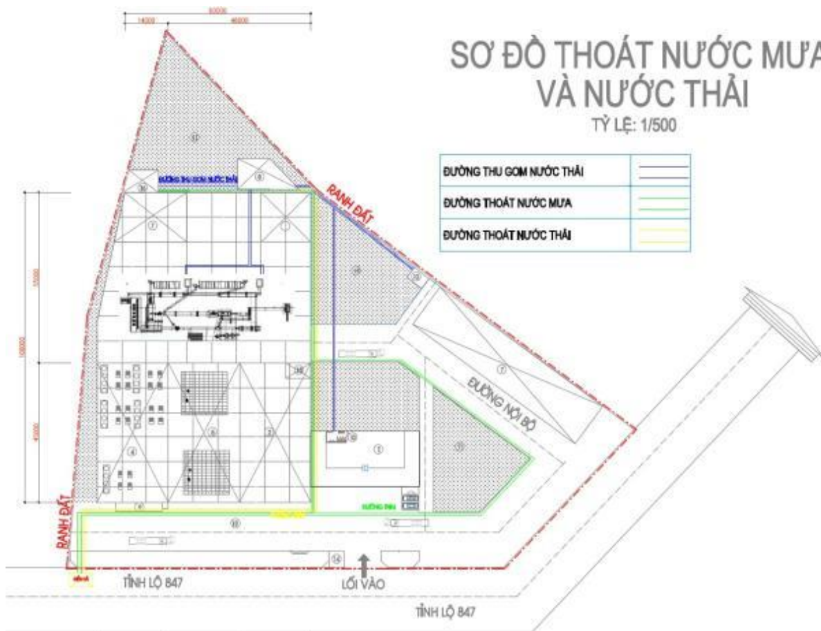
Hình 4.1. Sơ đồ mạng lưới thoát nước mưa và nước thải của Nhà máy
