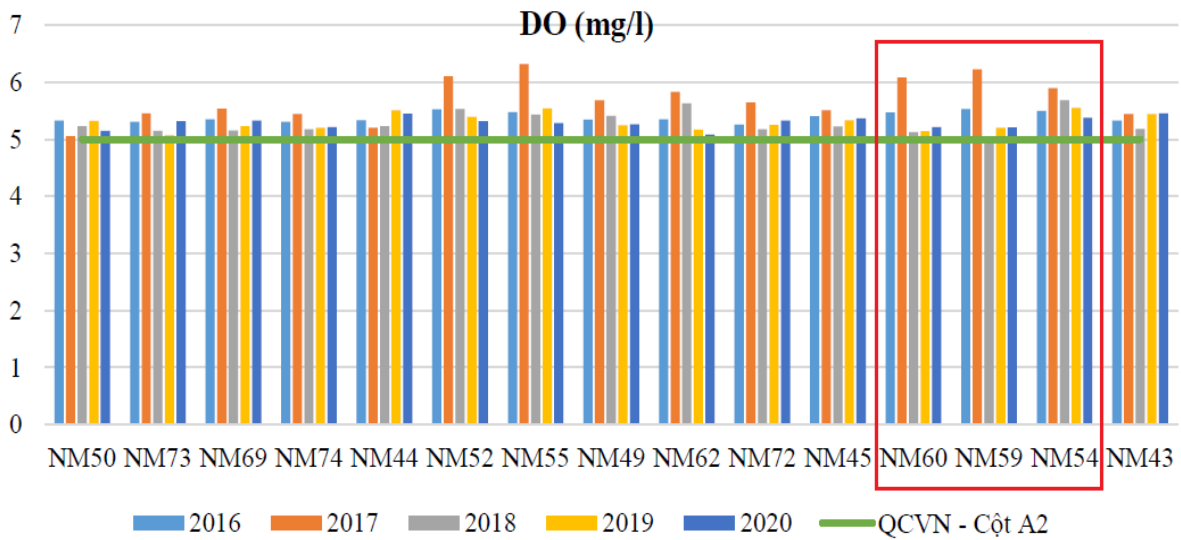
Diễn biến thông số DO của nước mặt trên sông Tiền, gần khu vực dự án
