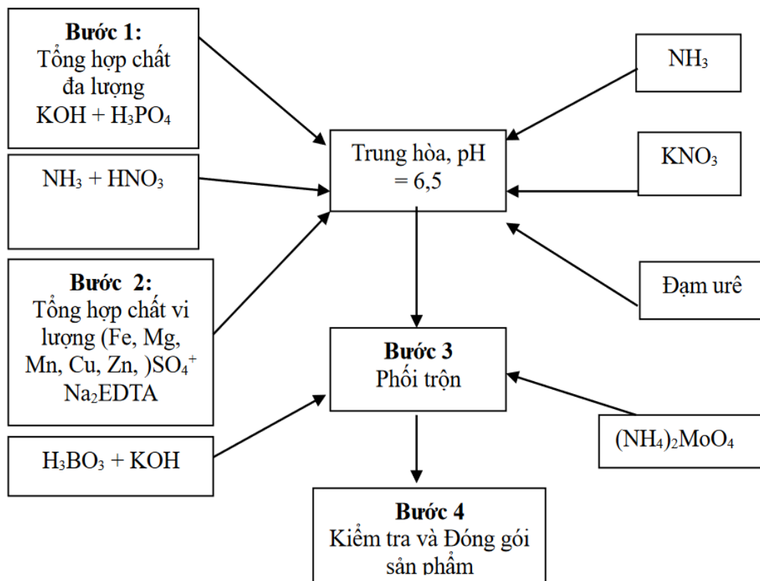
Hình 1.4. Quy trình công nghệ sản xuất phân bón NPK dạng lỏng
